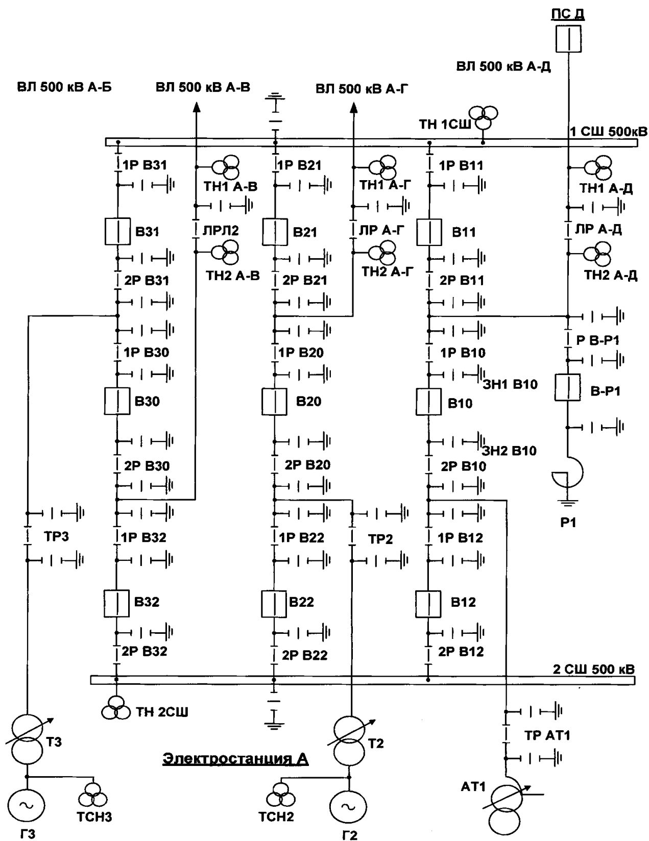
Рисунок 4. Полutorная схема РУ
